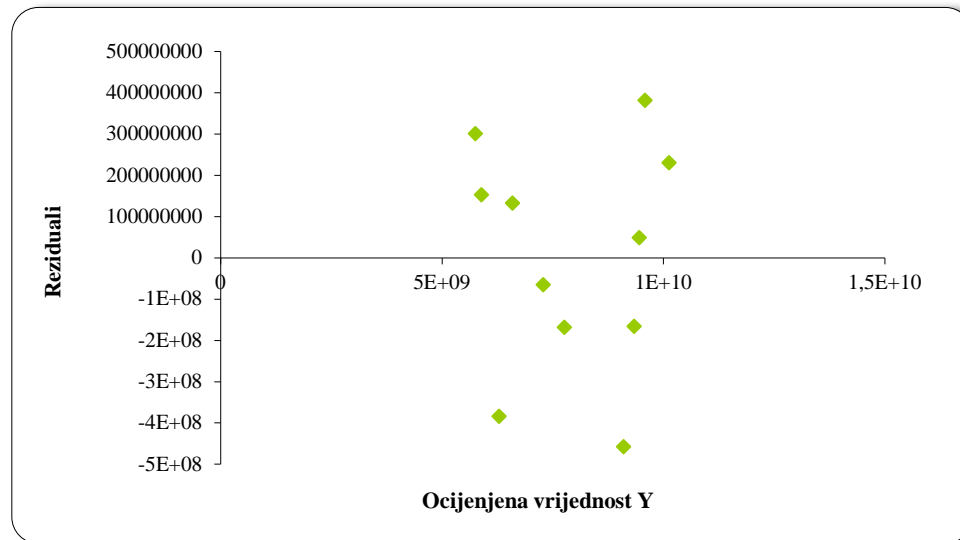
Grafikon 45: Grafičko utvrđivanje prisutnosti heteroskedastičnosti u drugom segmentu modela
