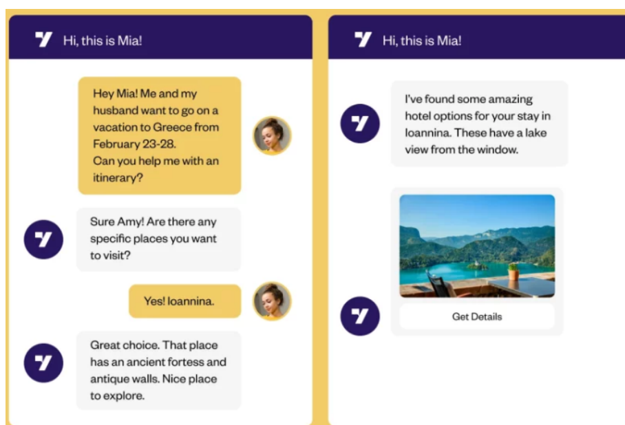
Slika 2. Primjer chatbotova
